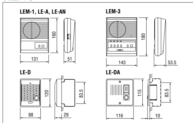
LEM-1;铃声或语音。LEM-3;具有铃声或语音的选择性呼叫。分机有铃声和LED显示
