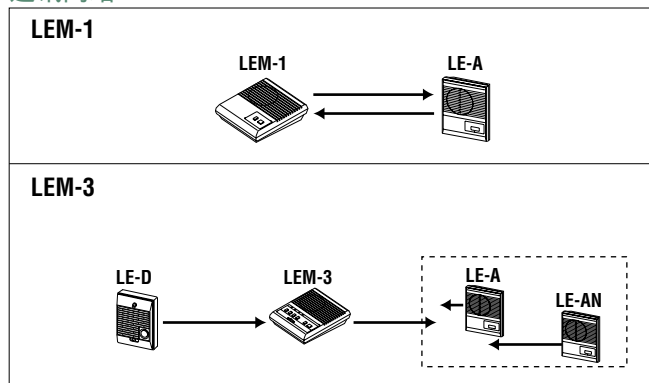
LEM-1;铃声或语音。LEM-3;具有铃声或语音的选择性呼叫。分机有铃声和LED显示
