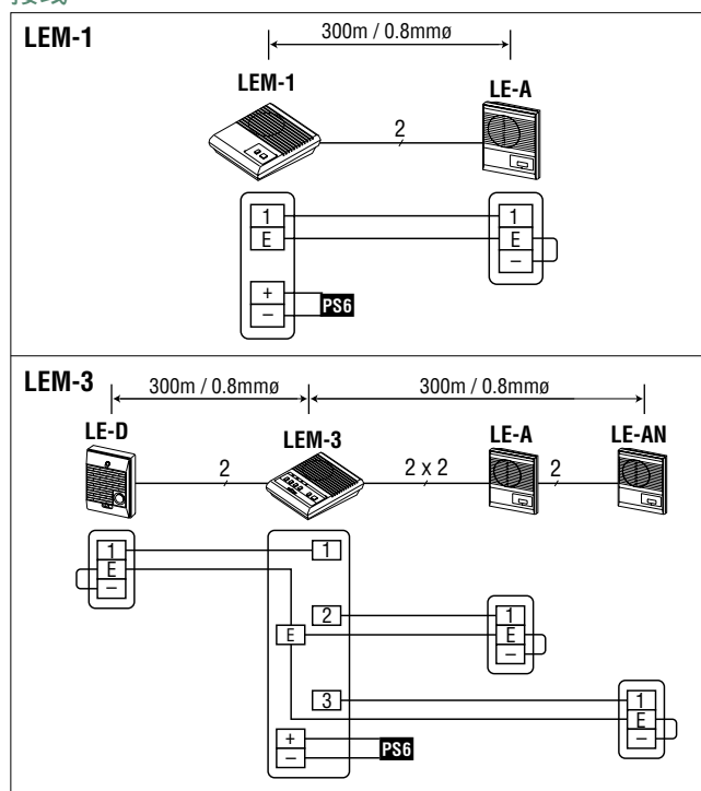
★ 不要拆除分机上的短路连接线。 PS6 : PS-0602D, PS-0602C
